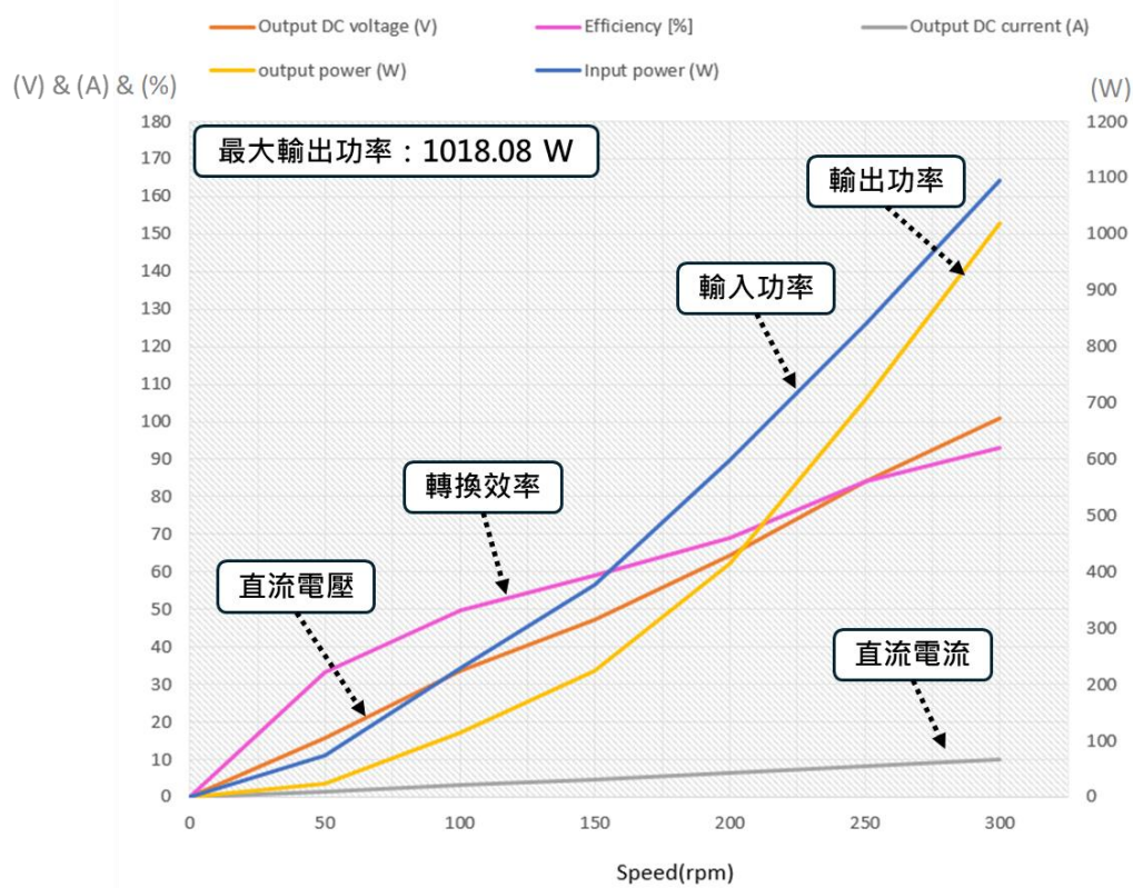
圖 21 Halbach AFPM 發電機性能曲線（海爾貝克排列）
