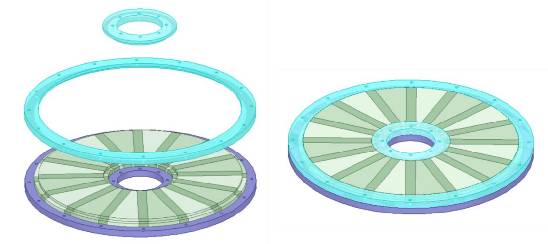
圖 5 轉子線圈爆炸圖 (合併)
