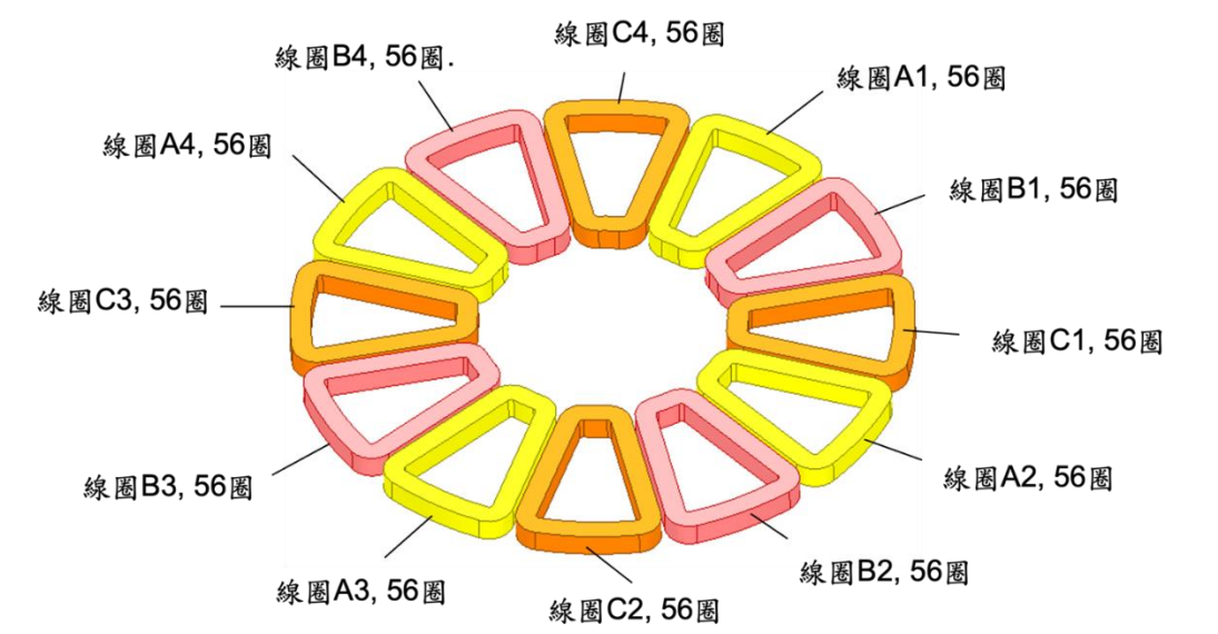
圖 4 線圈排列圖
