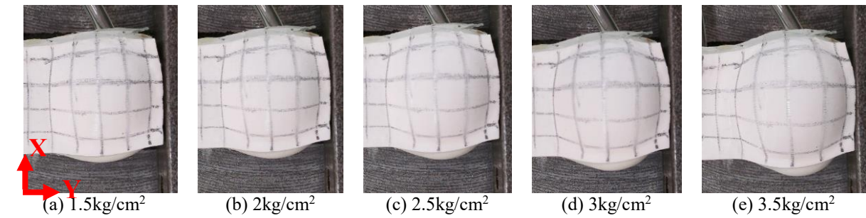
圖 8 氣囊變形觀察實驗設計，以一組實驗為例
