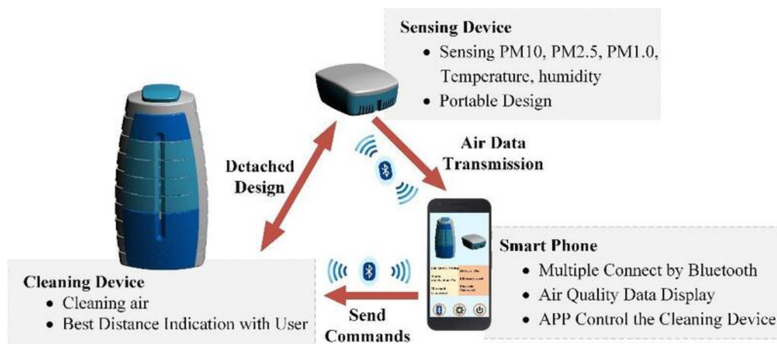
圖 1 系統架構圖
