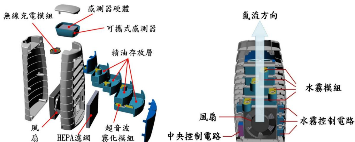
圖 6 空氣清新裝置結構與元件配置側視圖、後視圖
