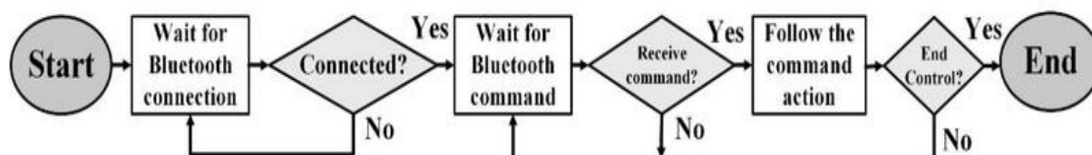
圖 3 空氣清新裝置流程圖
