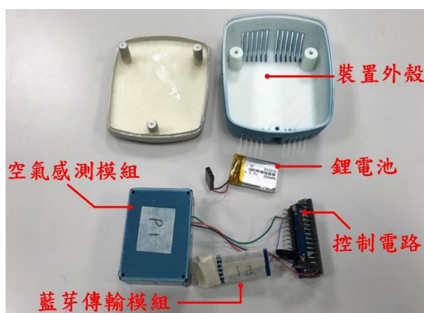
圖 7 空氣感測裝置內部元件圖
