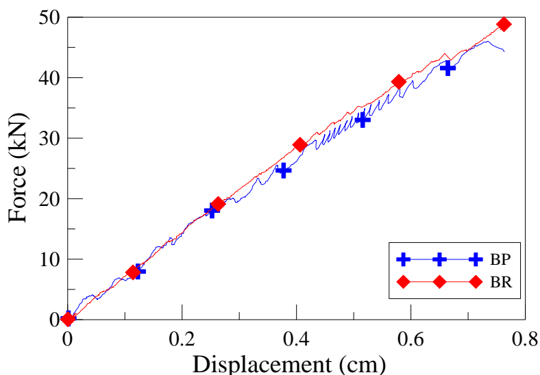
圖 7 BP 及 BR 梁構件受彎矩及剪力變形之力-位移關係圖
